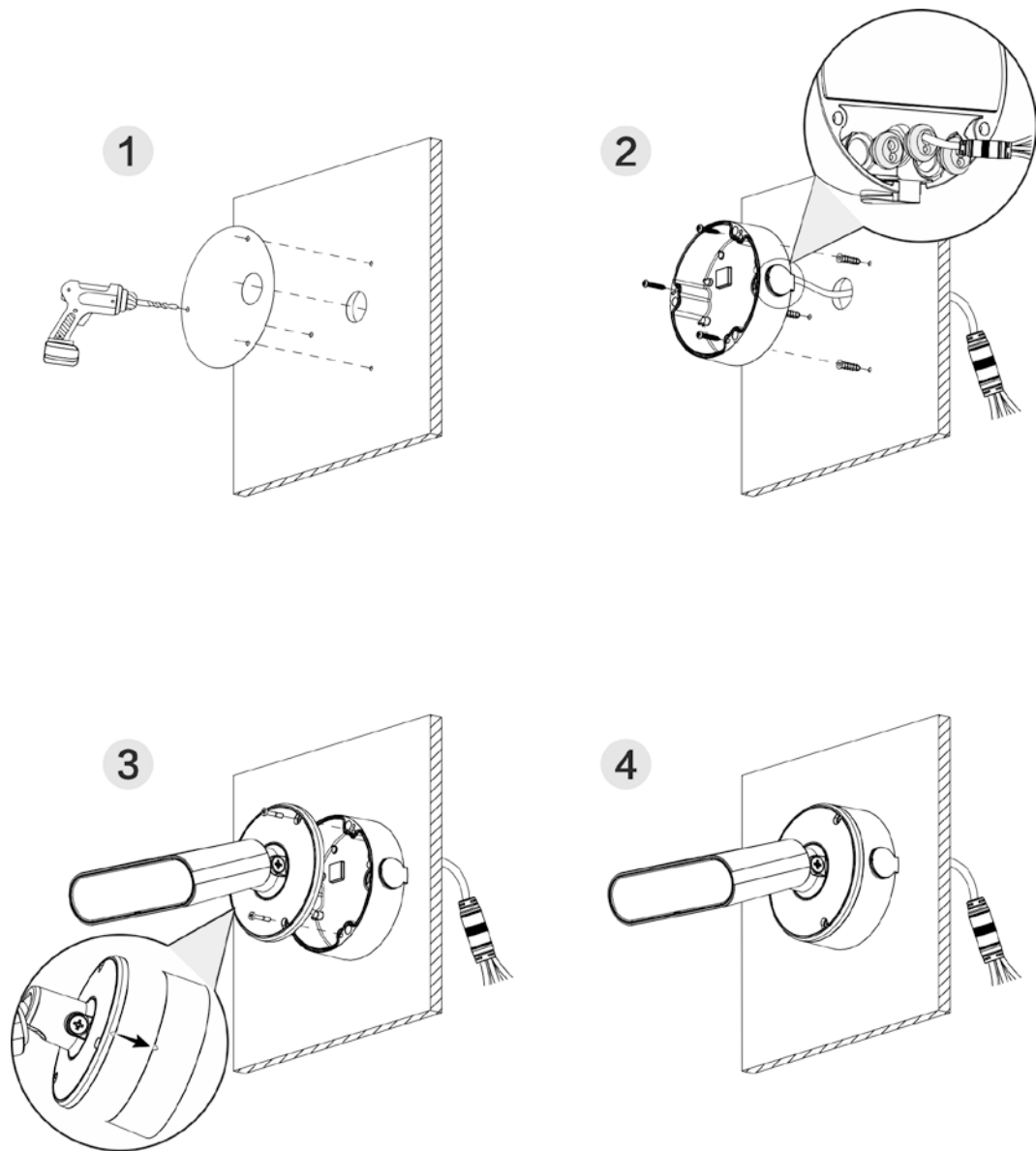
图3-5 墙体出线安装示意图
