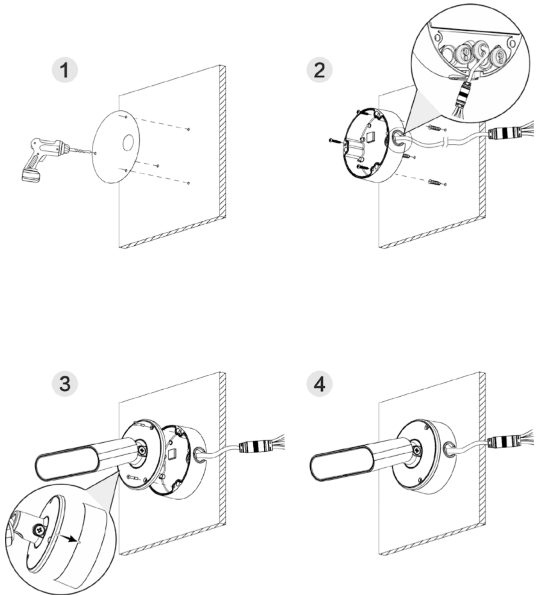
图3-6 出线槽出线安装示意图
