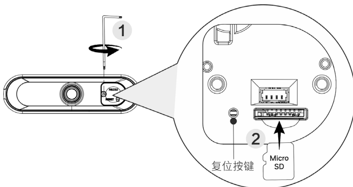
图3-4 安装 SD 卡示意图
