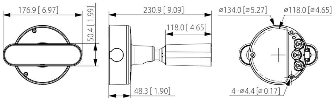
图3-2 结构尺寸示意图
