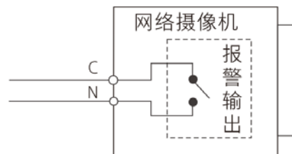
图1-3 报警输出示意图
